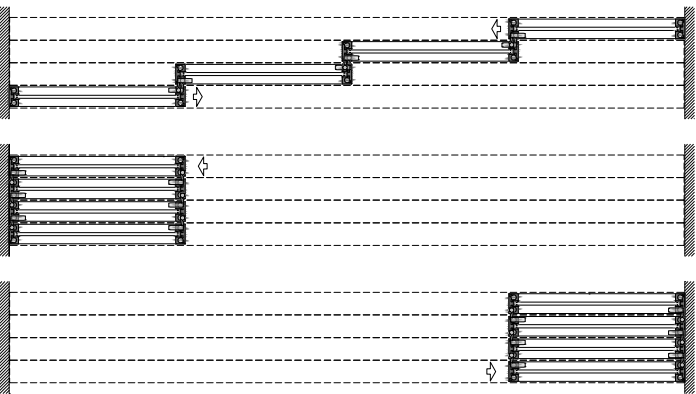
BINARIO A SOFFITTO A 4 VIE / 4 WAY CEILING TRACK
