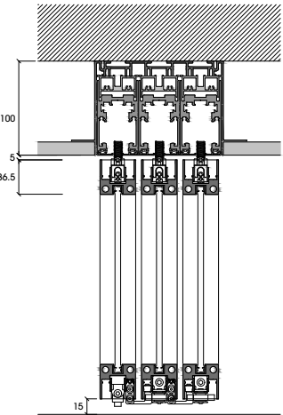
SEZIONE VERTICALE CON BINARIO A 3 VIE VERTICAL SECTION WITH 3 WAY TRACK
