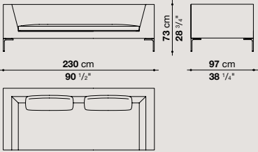
CH228
