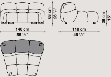
TY140CV_3
