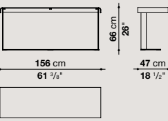
CHC156
