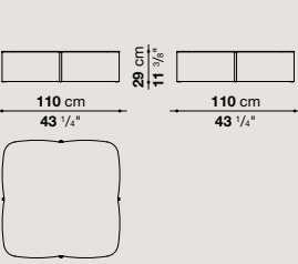
TYT110Q
