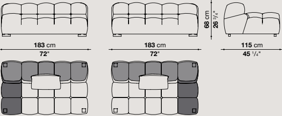
TY183BS_3 / TY183BD_3
