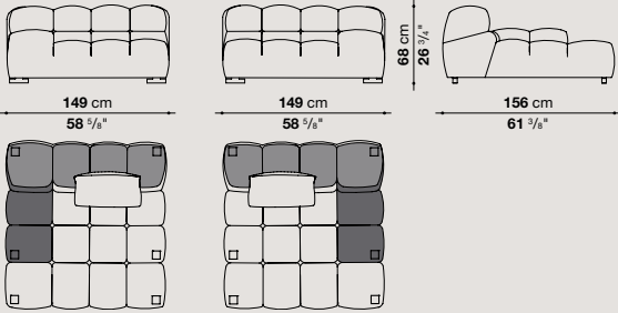
TY149BS_4 / TY149BD_4
