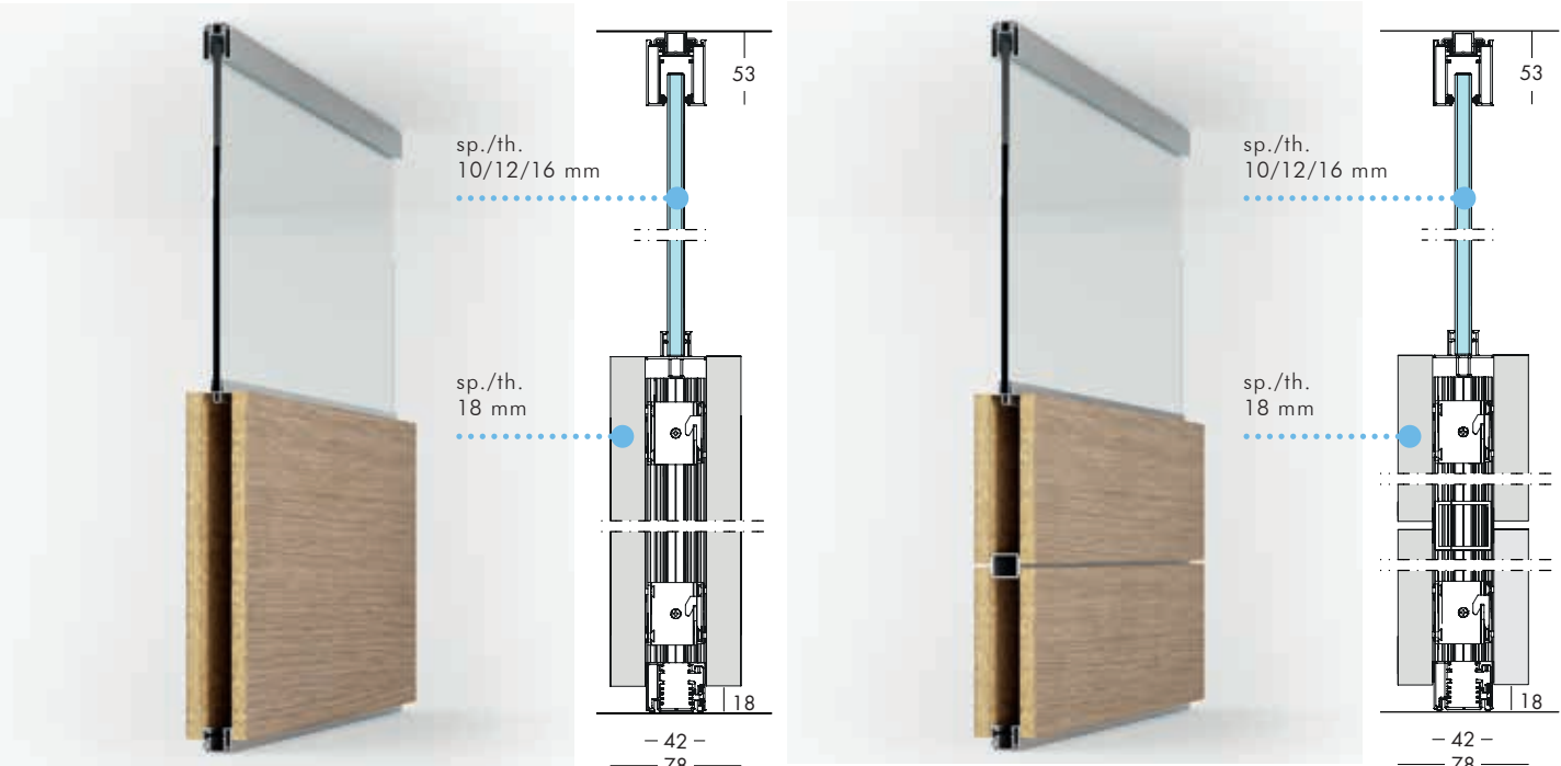
Parete divisoria mista Mixed partition wall Gemischte Wand Cloison mixte Mampara mixta
