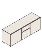
W./L. 1430 D/P. 442 H. 540 mm
