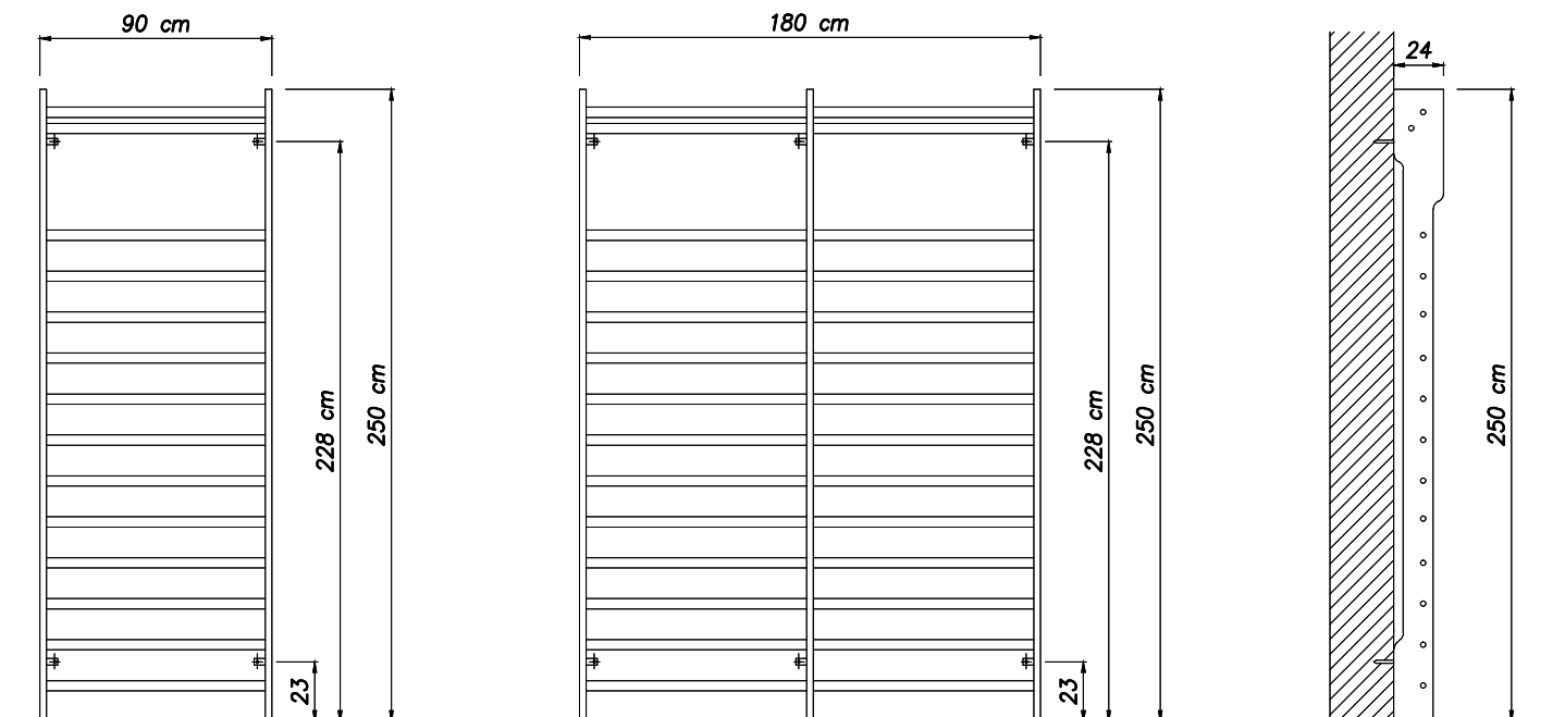
Art. 005362 Spalliera 1 campata
