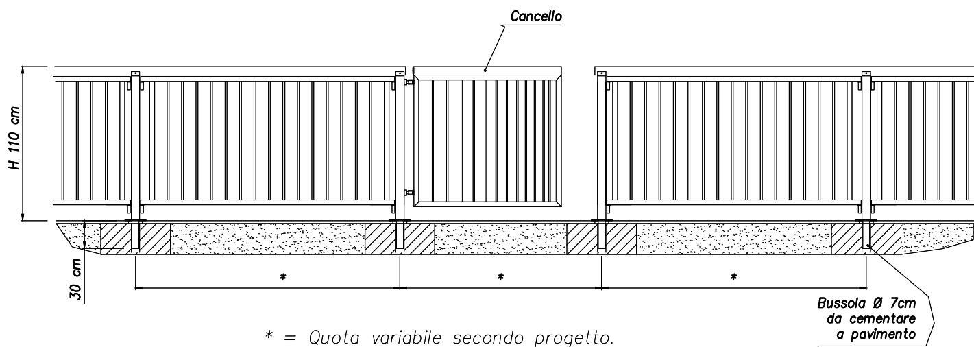
Art. 008610 Transenna su bussola
