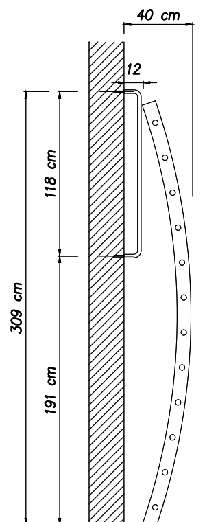
Art. 005280 Scala ortopedica curva
