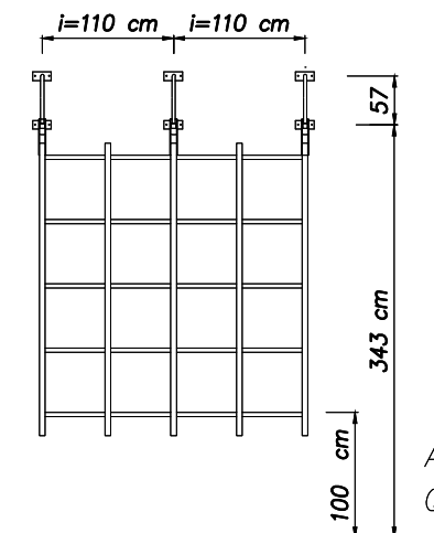
Art. 005251 Quadro svedese 36 fori
