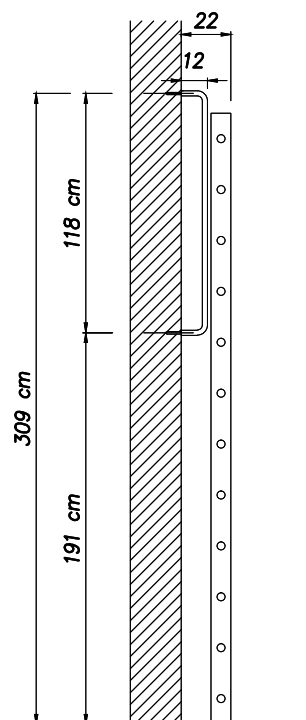
Art. 005270 Scala ortopedica diritta
