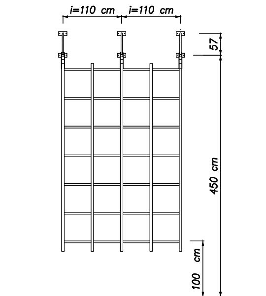
Art. 005241 Quadro svedese 24 fori
