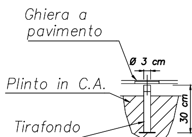
POSIZIONAMENTO TIRAFONDO PAVIMENTO GALLEGGIANTE
